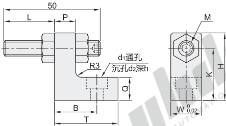
紧凑型限位块+定位螺栓 ICZ17/18
