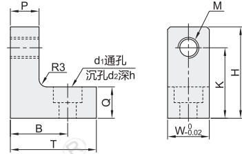
紧凑型限位块+聚氨酯螺钉 ICZ19/20
