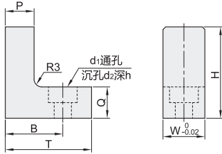
紧凑型限位块+定位螺栓 ICZ17/18
