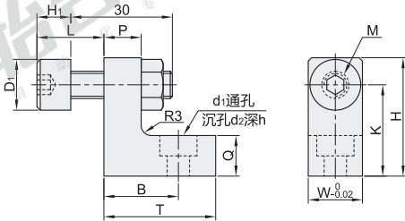
紧凑型限位块+聚氨酯螺钉 ICZ19/20
