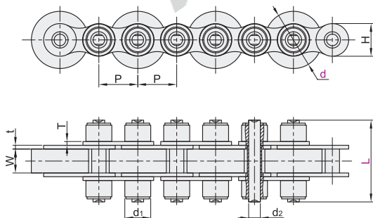
倍速链条 VMW21/22/23
