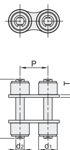
倍速链条接头 VMV83/94/95
