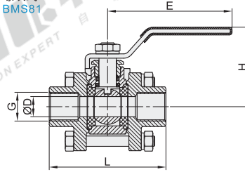
螺纹式 BMS81
