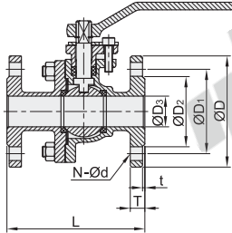
法兰式 BMS80
