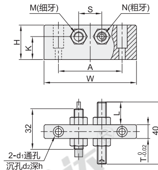
方型限位块+缓冲调节 ICR83/84/85
