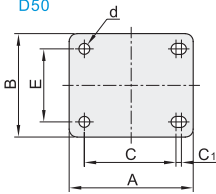
安装面 D50
