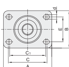
安装面 J-CRB16-D75
