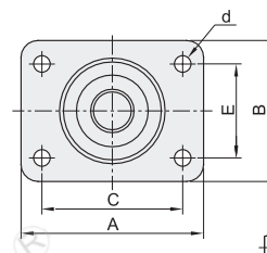
安装面 J-CRB16-D75A/D75B
