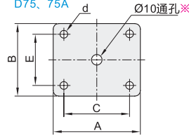
安装面 D75、75A
