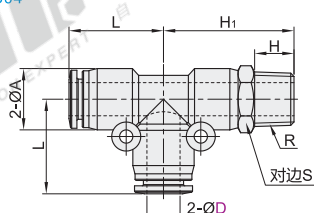
T型侧三通接头 XZS04
