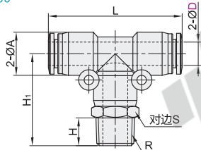
T型三通接头 XZS03
