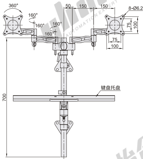
安装板尺寸
