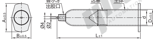
卡口带弧型 BMM37
