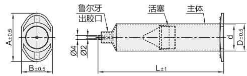
卡口直线型 BMM38
