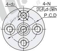
圆法兰型
