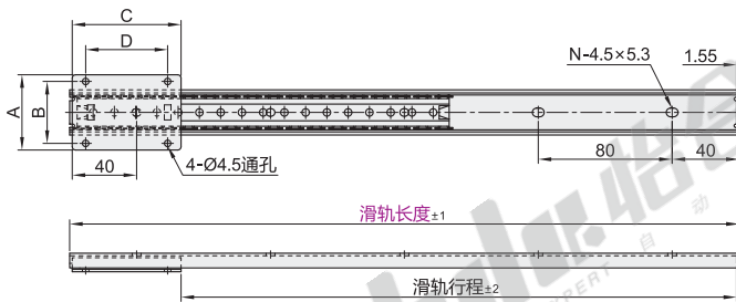
通孔 IDD06
