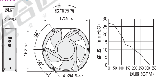
外形尺寸：172
