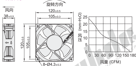
外形尺寸：12038
