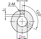
(键槽+螺孔型) N
