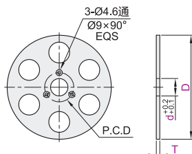
锥孔型(A6061) ZCH73/74
