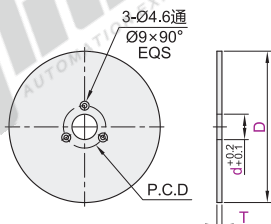
锥孔型(有机玻璃) ZCH72
