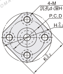
方法兰 E-BFF61/62/63/64/66
