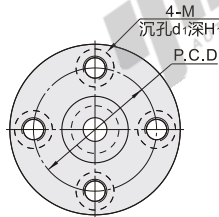
圆法兰 E-BFF51/52/53/54/56
