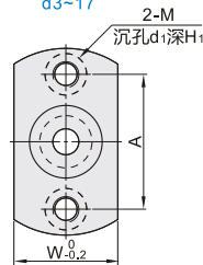
对边法兰 E-BFF71/72/73/74/76
