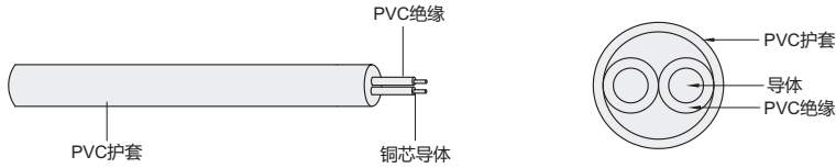
RVV聚氯乙烯绝缘聚氯乙烯护套软电缆
