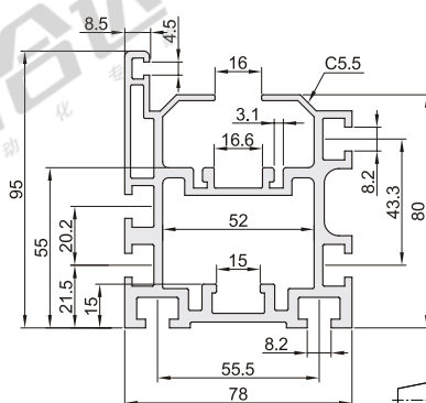
ATS05-25-31DG (此型号需另外采购钢轨)
