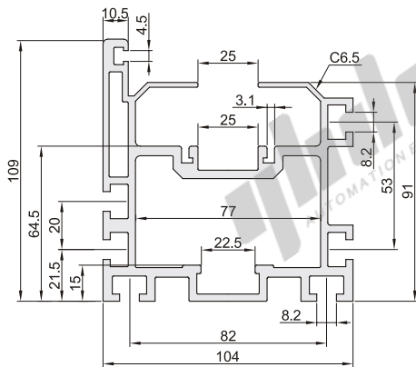
ATS05-30-38DG (此型号需另外采购钢轨)
