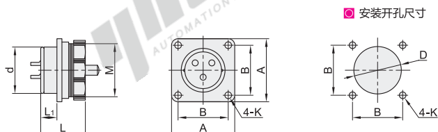
安装开孔尺寸
