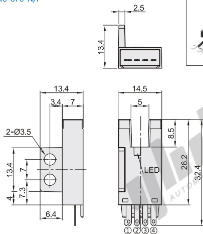
ZJF40-676-N/P F型
