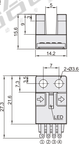
ZJF40-677-N/P R型
