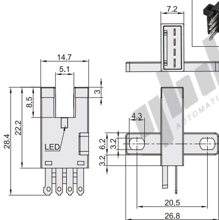
ZJF40-672-N/P T型
