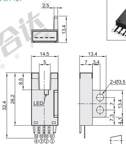
ZJF40-677-N/P R型
