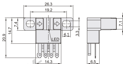
ZJF40-674-N/P Y型
