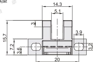
ZJF40-671-N/P L型
