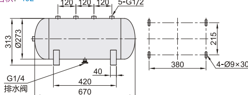
容积：40L
