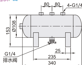
底架安装孔尺寸
