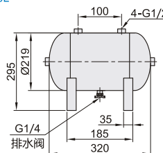
底架安装孔尺寸
