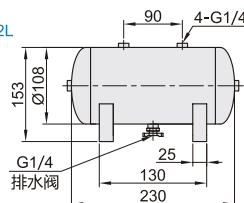
底架安装孔尺寸
