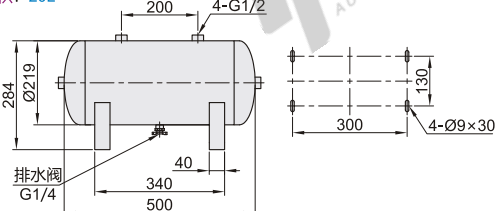
容积：20L
