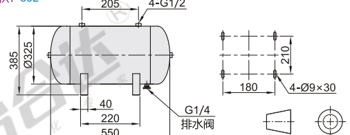
容积：50L
