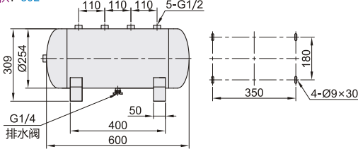
容积：30L
