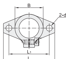
长导向型 GFC11
