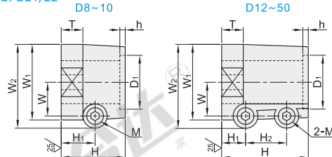
长导向型 GFD21/22
