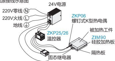
24V电源接线示意图
