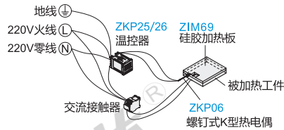
220V电源接线示意图
