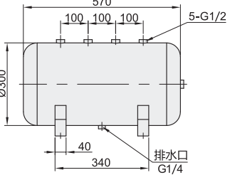
底架安装孔尺寸
