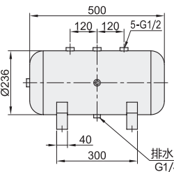
底架安装孔尺寸
