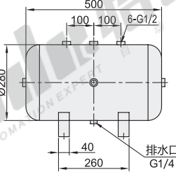
底架安装孔尺寸
