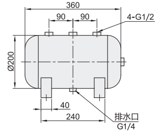
底架安装孔尺寸
