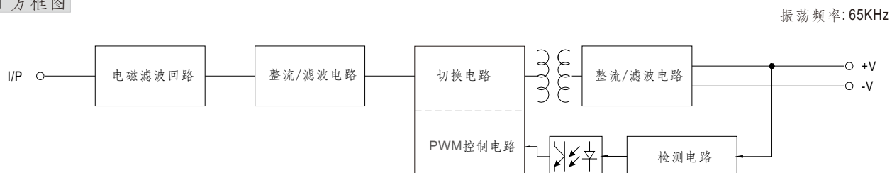
■ 方框图
