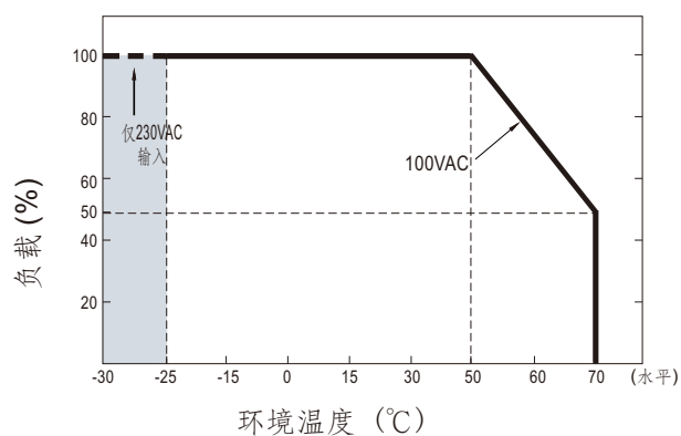
■ 减额曲线
