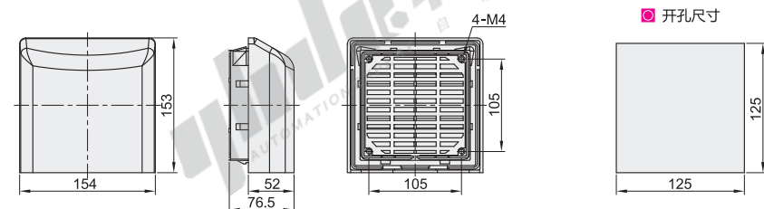
适用风扇尺寸: FY9803
