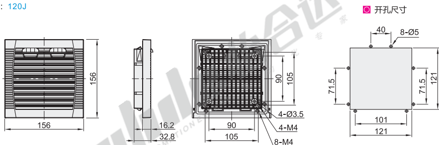
适用风扇尺寸: 120J
