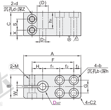
偏置型 RCG21/22
