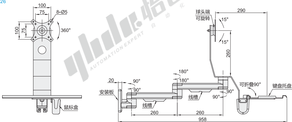
安装板尺寸
