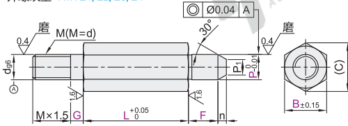
外螺纹型 YMY21/22/23/24
