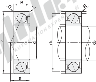
安装图
