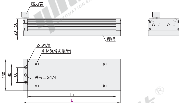
海绵式 WEY81
