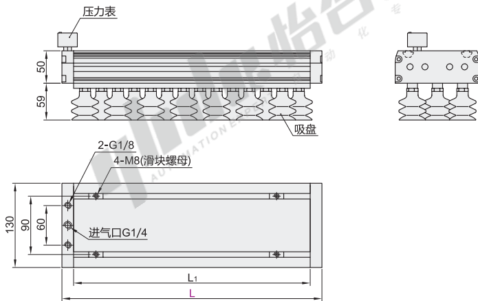
吸盘式 WEY82
