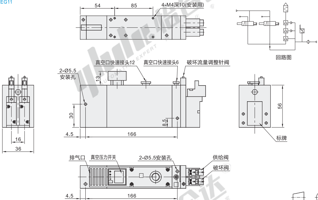
带真空压力开关、带阀组合 WEG11
