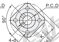
方法兰型 GAJ11/12/16
