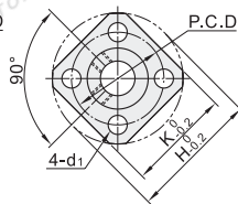
方法兰型 GAC11/12/16/18/19
