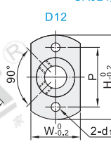
对边法兰型 GAJ21/22/26
