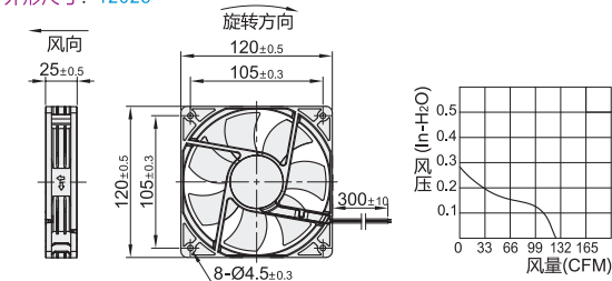
外形尺寸：12025
