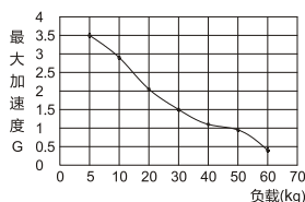
最大加速度VS负载
