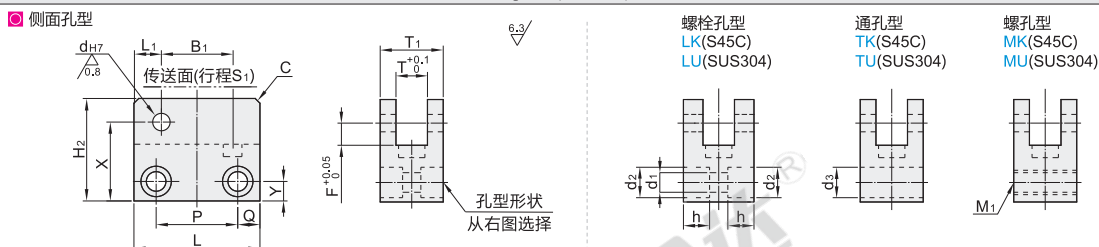
③底座(详细尺寸)
