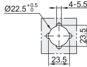
开孔尺寸
