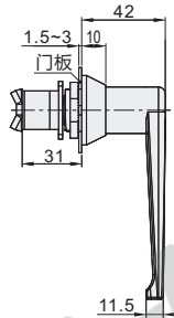
安装方向
