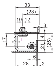
安装尺寸图
