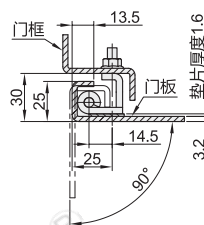
90°打开时
