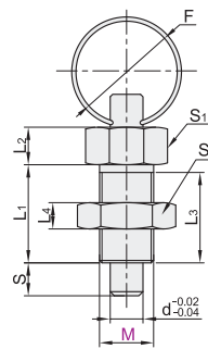
带锁紧螺帽 ZAC43 ZAC44 ZAC45
