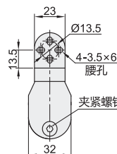
末端安装块选择 X(尼龙安装块)
