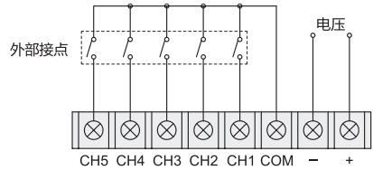
接线图
