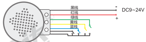
4路触发接线图
