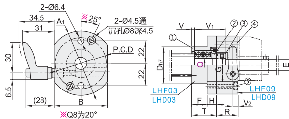
套装-支座固定侧+防转动固定件 (适用小型数字式位置显示器) LHF22/LHD22
