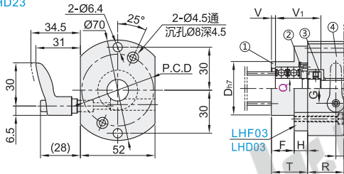
套装-支座固定侧+防转动固定件 (适用大型数字式位置显示器) LHF23/LHD23
