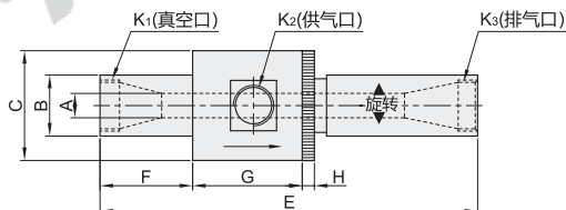
吸入流量可调型 WEC81
