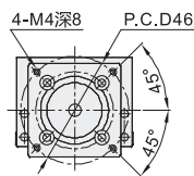
马达连接 支座: F3
