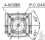
马达连接 支座: F2
