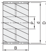
斜齿(右旋) VNQ12
