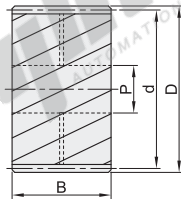
斜齿(左旋) VNQ11
