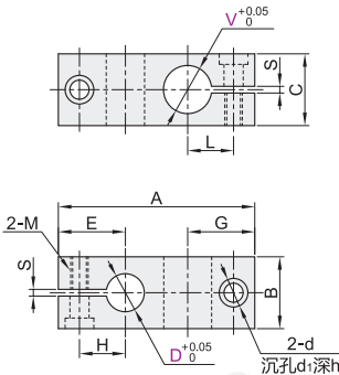
异径直交型 RDN11/12
