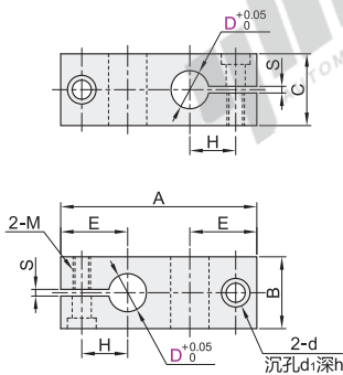
同径直交型 RDN01/02
