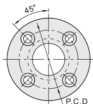
标准型 WHL01/02
