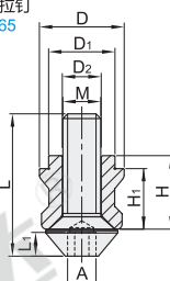
夹紧拉钉 ZFH65
