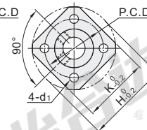
方法兰型 GAJ11/12/16
