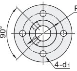
圆法兰型 GAJ01/02/06
