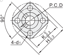
方法兰型
