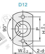
对边法兰型 GAJ21/22/26
