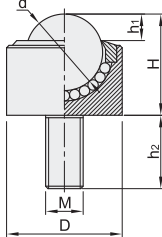
标准型 QFB11/12
