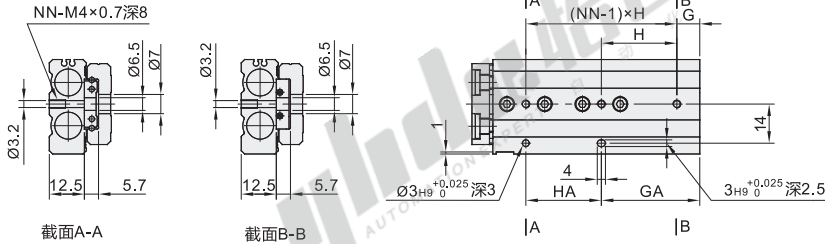
截面A-A
