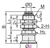
固定式顶部真空端口 J-WES61/62
