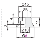
盘径Ø20
