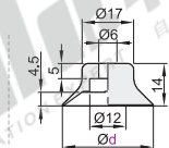
盘径Ø30
