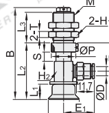
弹簧式侧面真空端口 J-WES71/72
