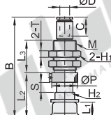
弹簧式顶部真空端口 J-WES66/67
